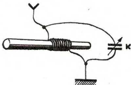
Rys. 3. Instalacja usprawniająca działanie aparatu. K — kondensator obrotowy
